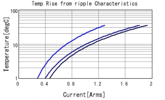
GCM188R71H104KA57 Temp. rise — 400kHz — 800I
