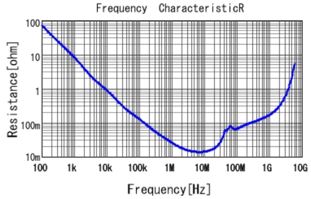
GCM188R71H104KA57 R DCOV, 25degC
