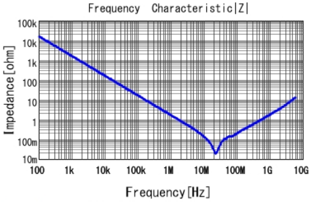
GCM188R71H104KA57 |Z| DCOV, 25degC
