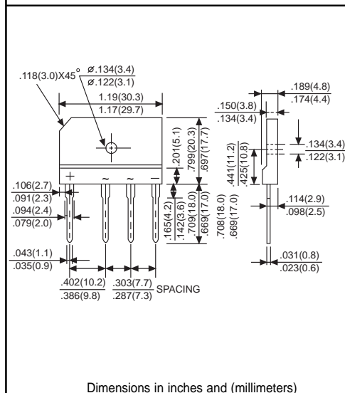
GBK
