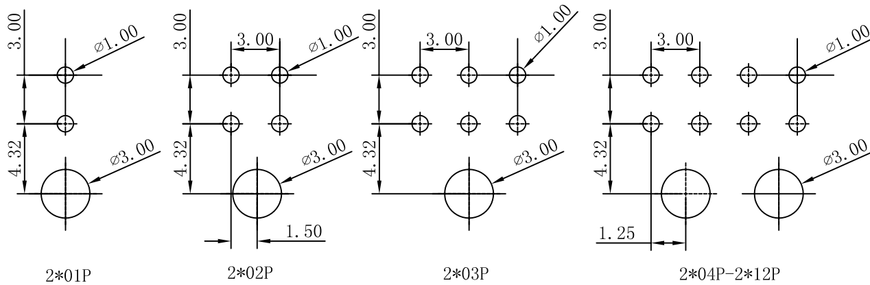
P. C. B. LAYOUT
